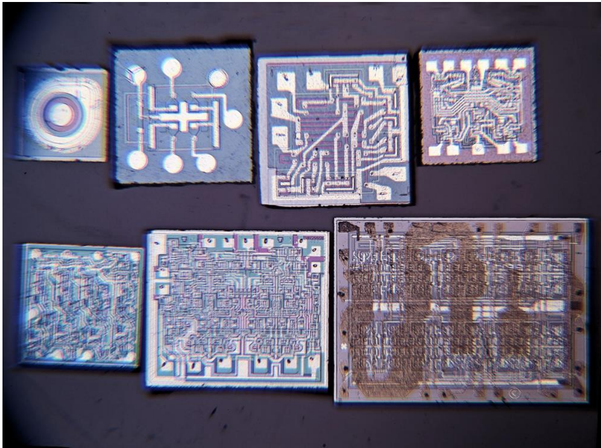
Figura 2 - Fotografias dos 5 dispositivos usados por Gordon Moore para estabelecer a taxa de crescimento do número de componentes por chip. Os 2 maiores foram usados para verificar se a tendência de crescimento se mantinha. Estes dispositivos semicondutores foram fabricados pela Fairchild: transistor 2N697 (1959), \mu Logic Type G c/ 7 transístores (1962), \mu Logic Type R c/ 33 transístores (1963), DTL 945 c/ 34 transístores (1964), contador decimal C \mu L 958 c& 58 transístores (1964), 9300 registo de deslocamento de 4 bits c/ 125 transístores (1966), e Micromatrix 4500 conjunto de 32 portas lógicas programáveis c/ 264 transístores (1967). (Crédito: Computer History Museum)
