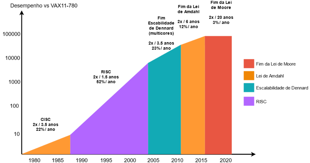
Figura 3 – Evolução do desempenho dos processadores ao longo dos últimos 50 anos. Crédito: John Hennessy and David Patterson, Computer Architecture: A Quantitative Approach , 6/e. 2018
